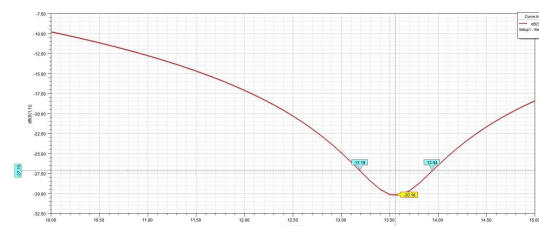
Figura 4: Frecuencia de resonancia y BW a -3dB.
