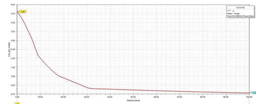
Figura 5: Campo magnético simulado en el centro del eje de la antena y a 10 cm sobre el mismo eje.
